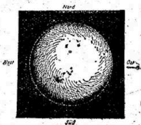
Fig. 4. Sonne mit Flecken.
