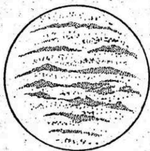
Fig. 18. Der Halley'sche Komet am 13. April 1910.
