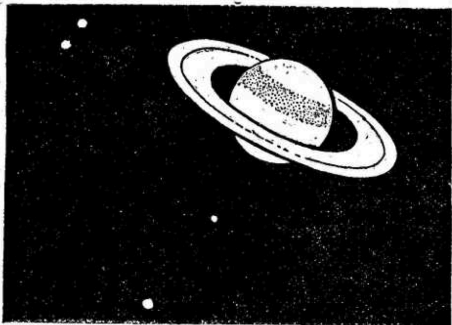
Fig. 17. Saturn mit Ring und vier Trabanten.
