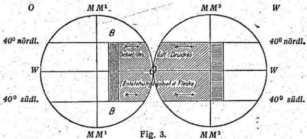
Umlaufsrichtung der Sonne bzw. des Mondes.
